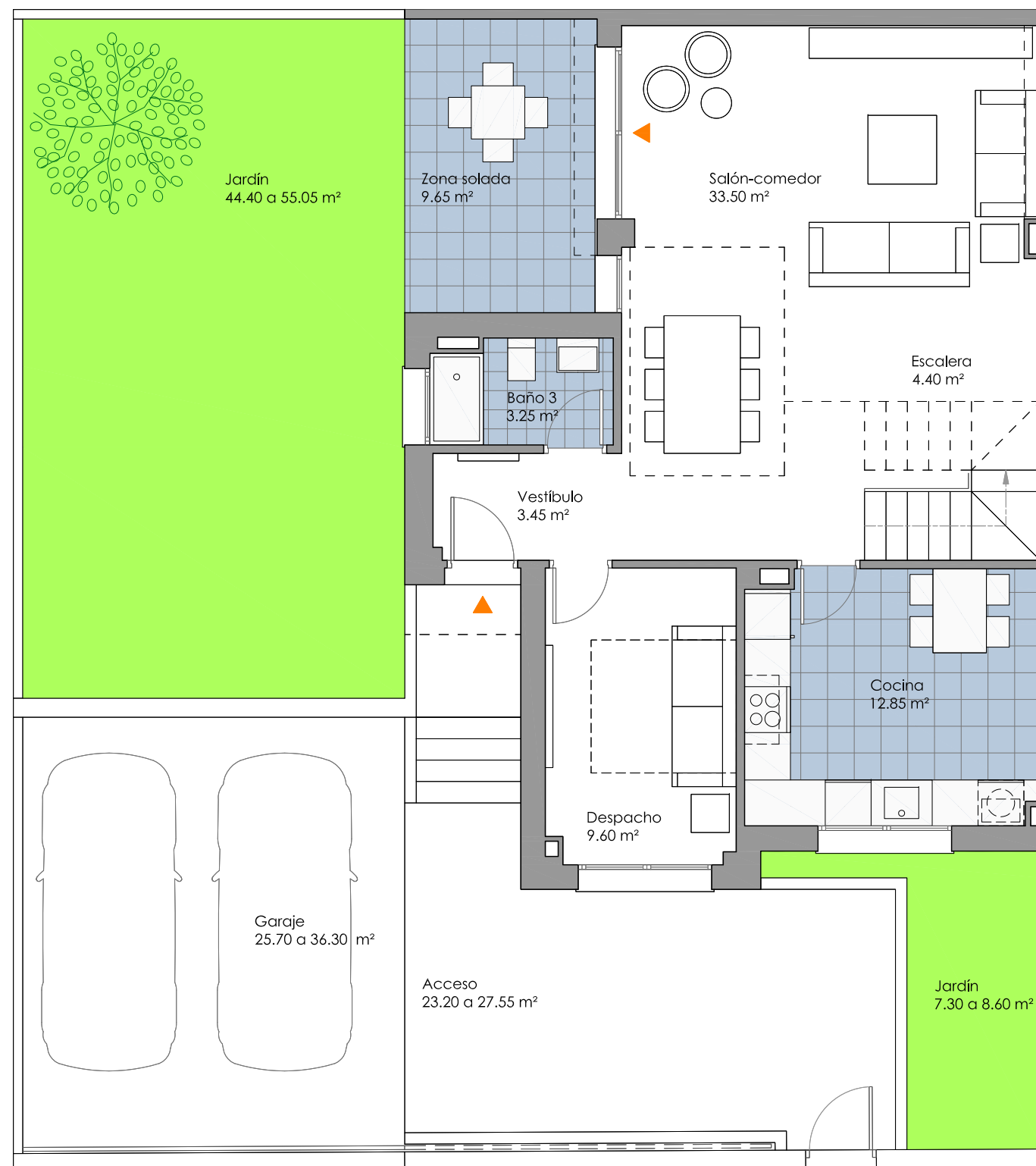
PLANTA BAJA
