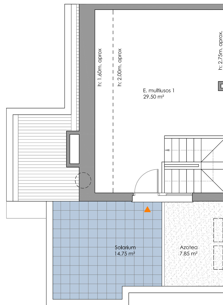
PLANTA BAJO CUBIERTA
