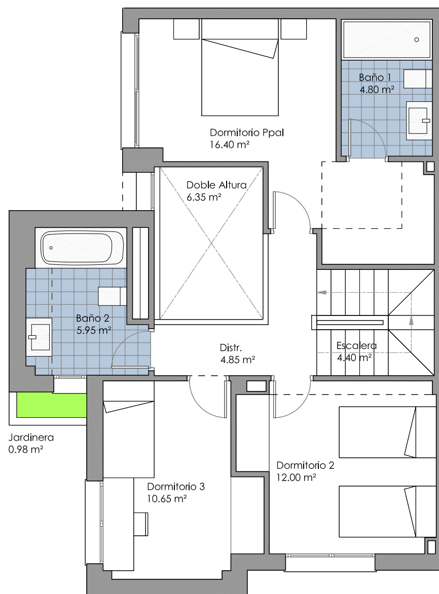
PLANTA PRIMERA
