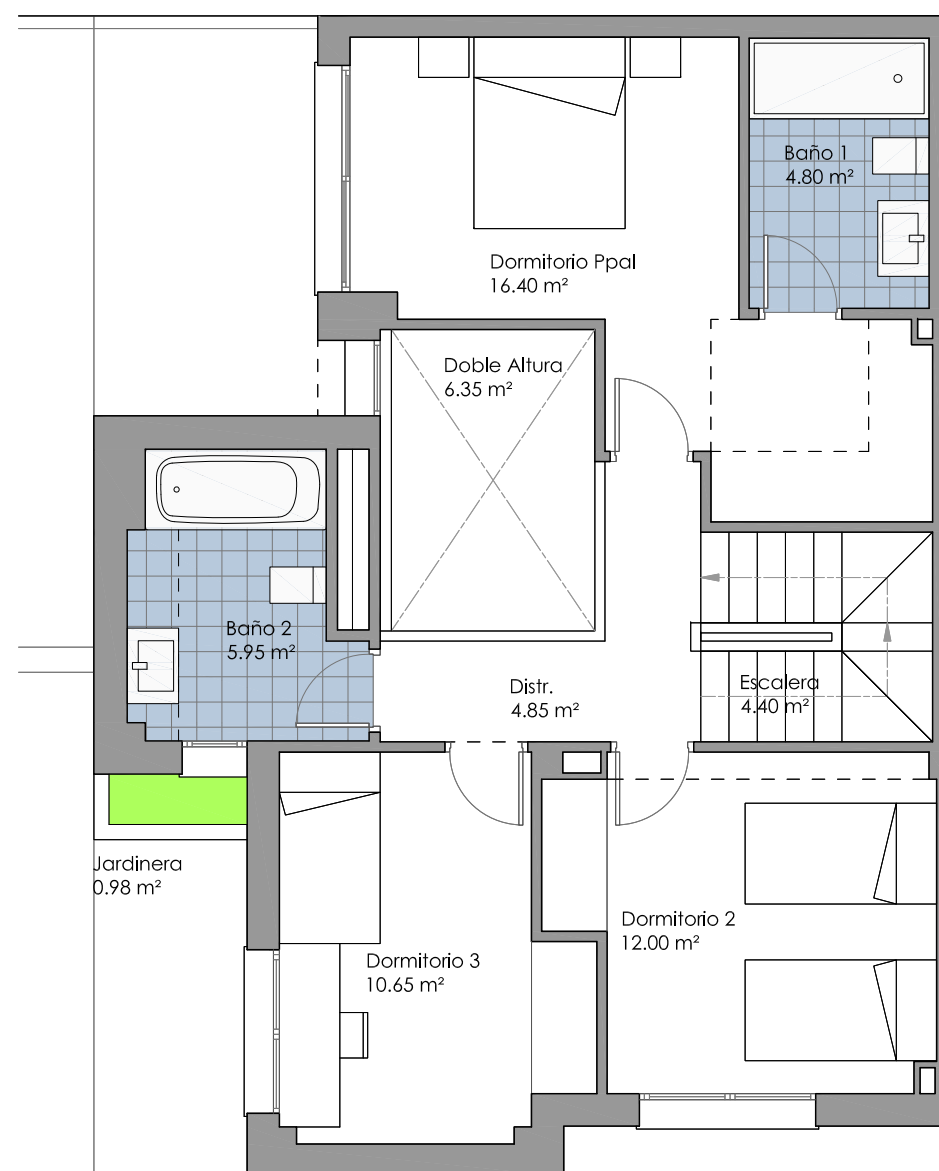
PLANTA PRIMERA
