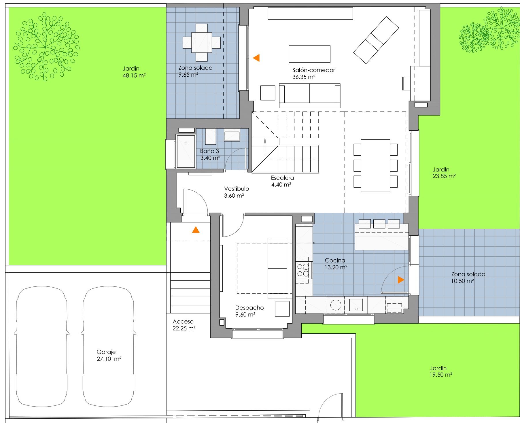
PLANTA BAJA
