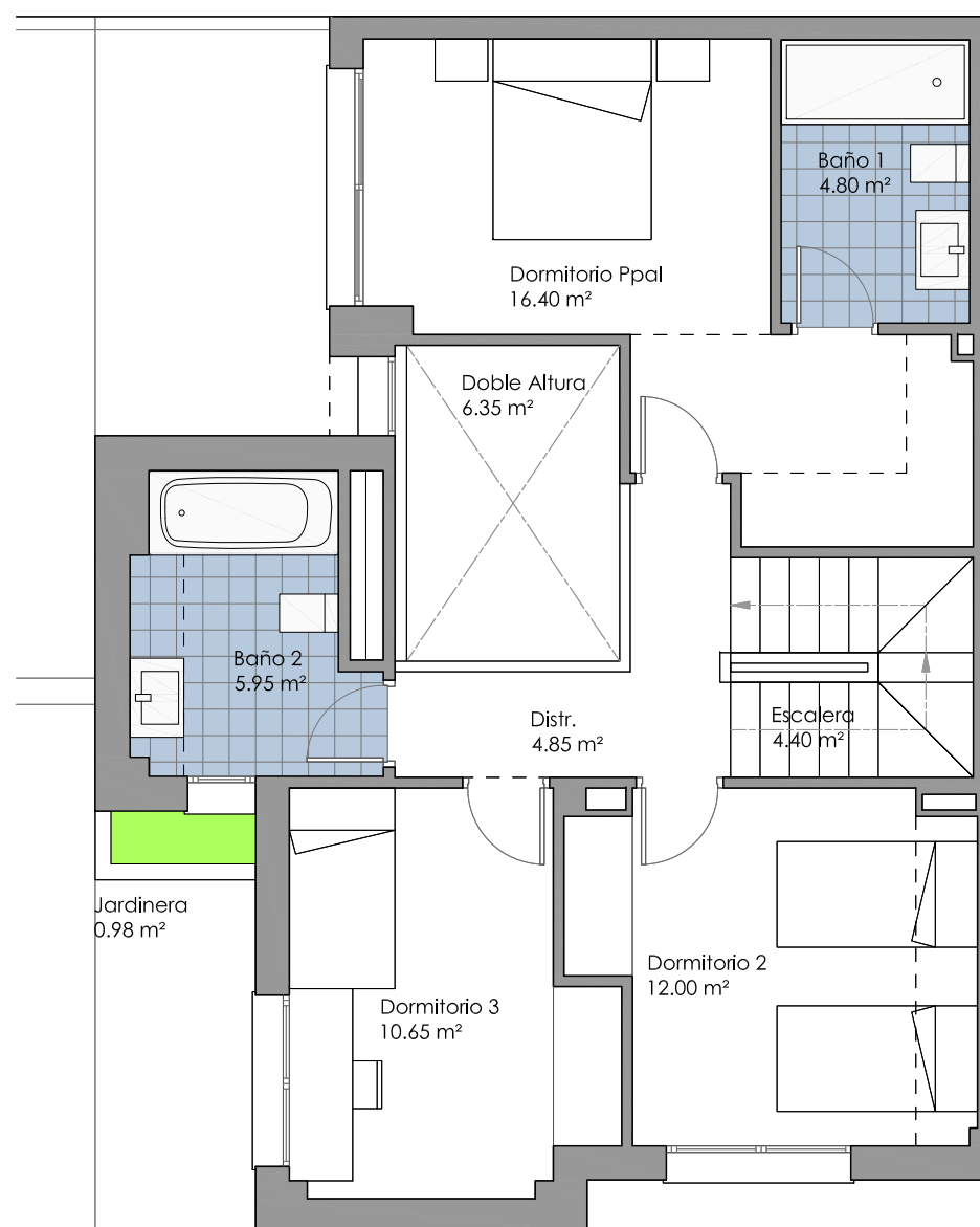
PLANTA PRIMERA
