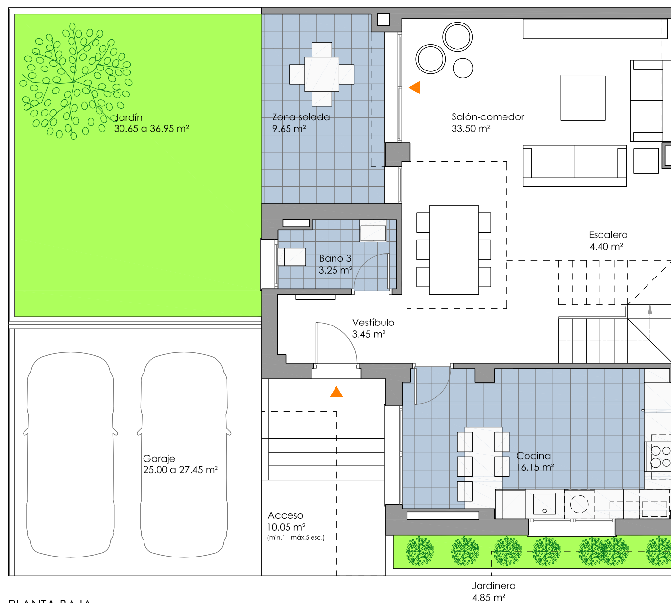
PLANTA BAJA
