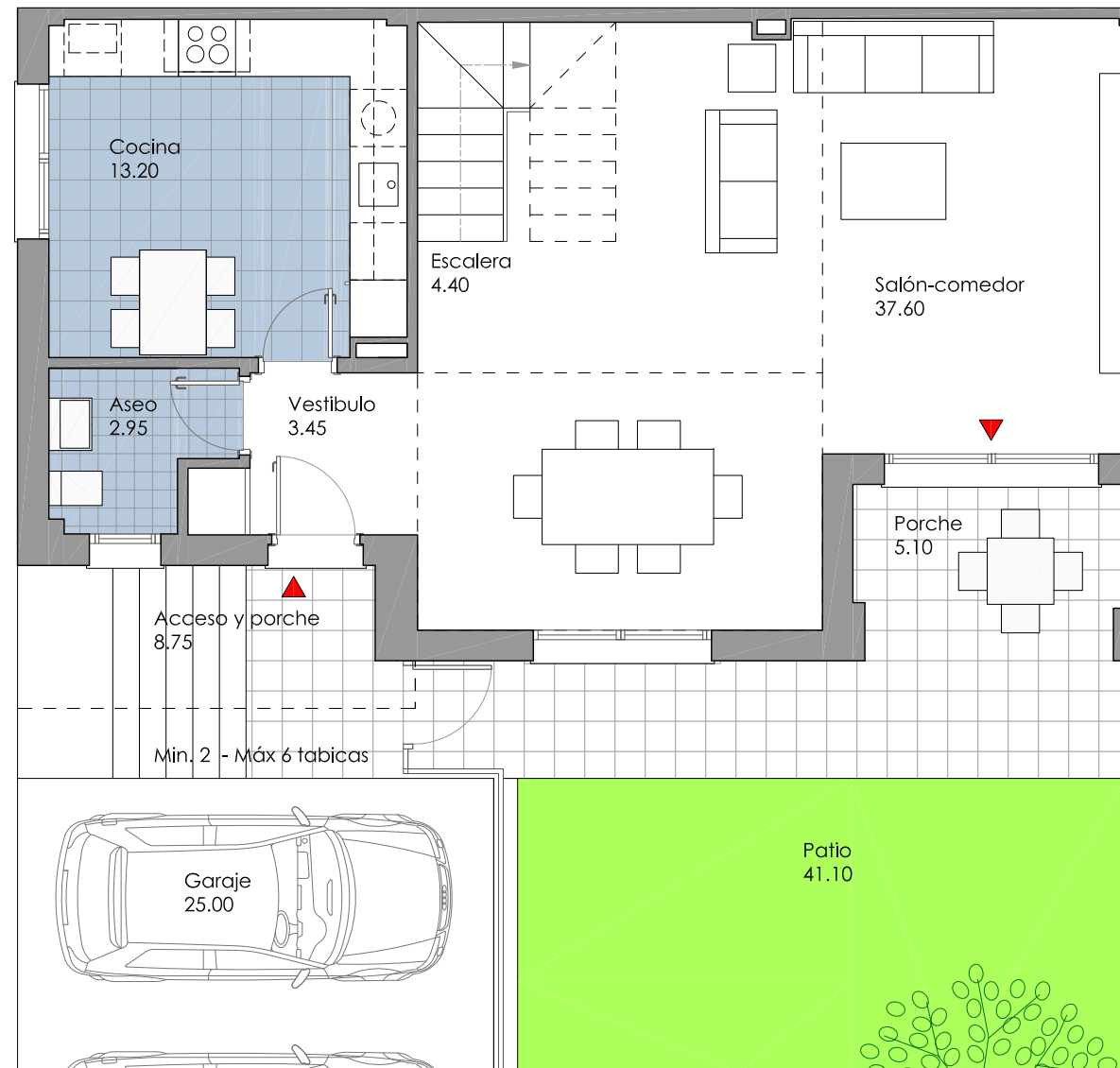
PLANTA BAJA
